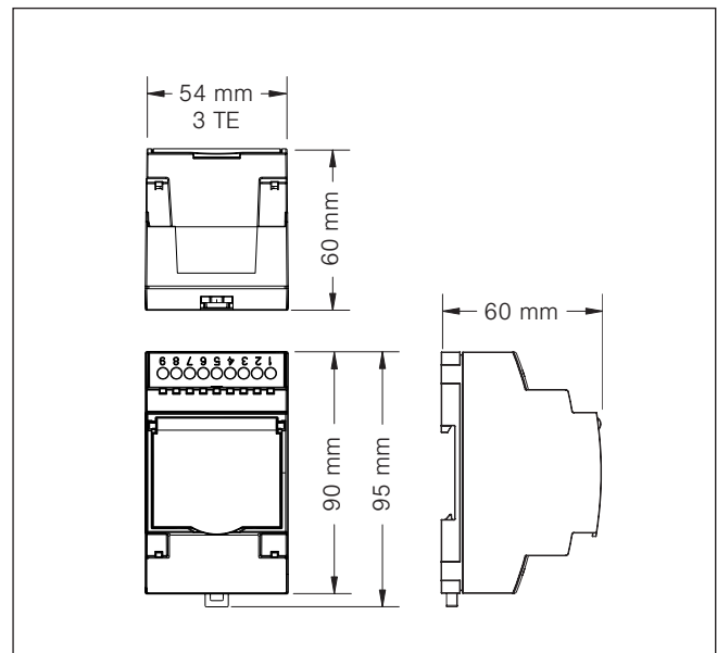
Abb. 4 Abmessungen
