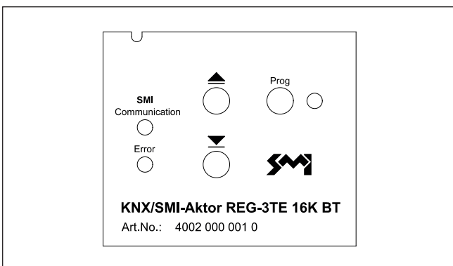
Abb. 3 Abdeckplatte
